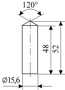
Şekil 2: Silindirik bronz piston, boyutları mm olarak
